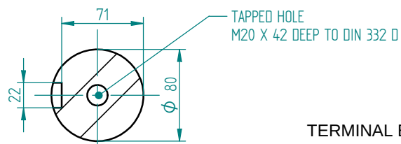
Przekrój A-A 1:3
