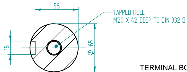
Przekrój A-A 1:2
