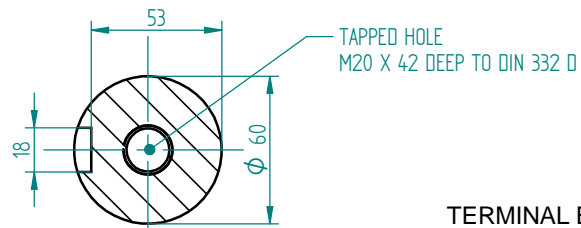
Przekrój A-A 1:2
